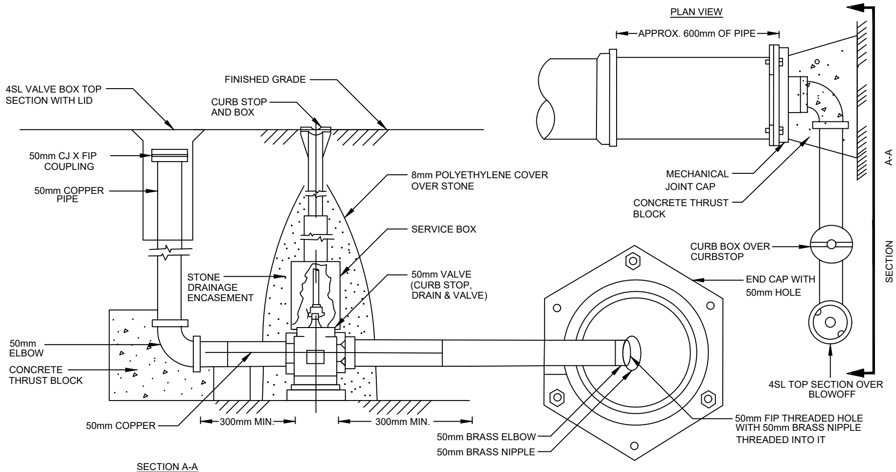
SECTION A-A
