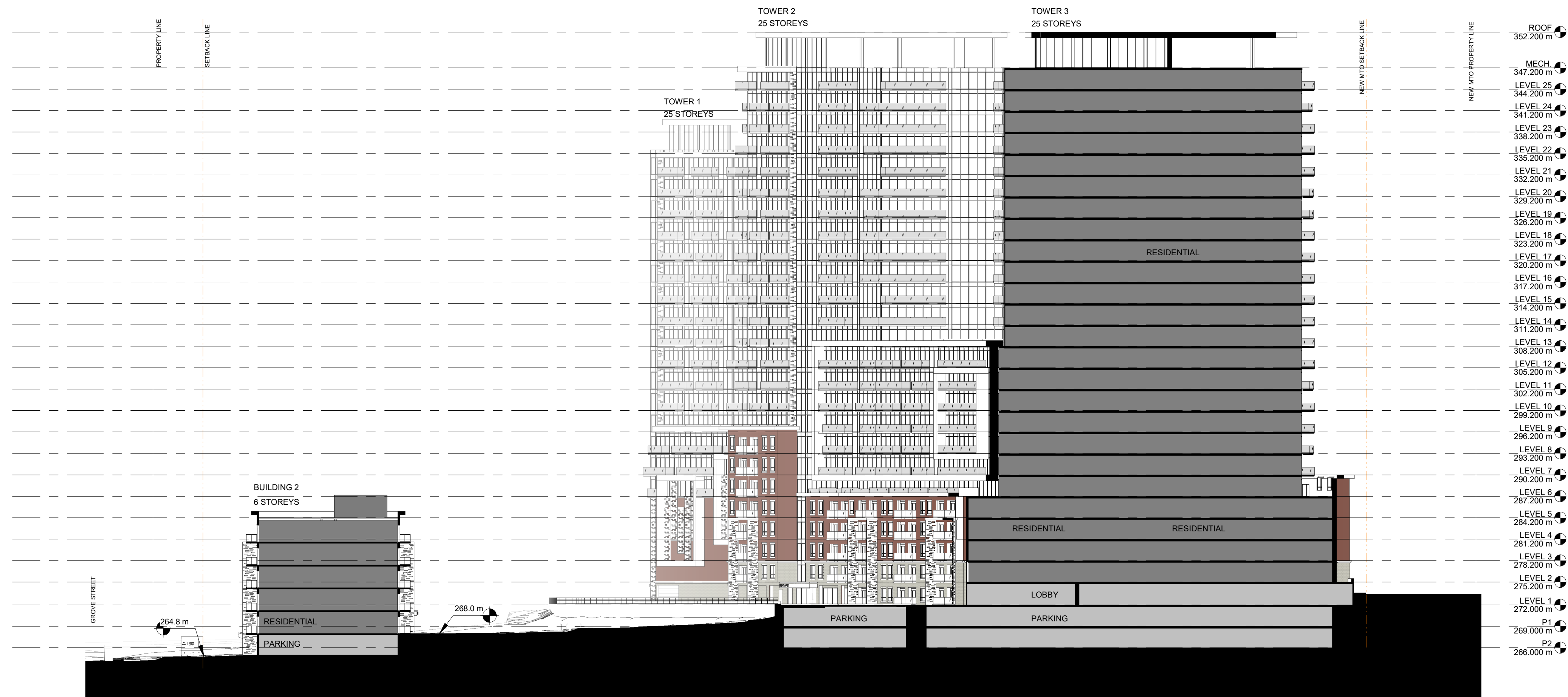
1 SITE SECTION 1 1:400
