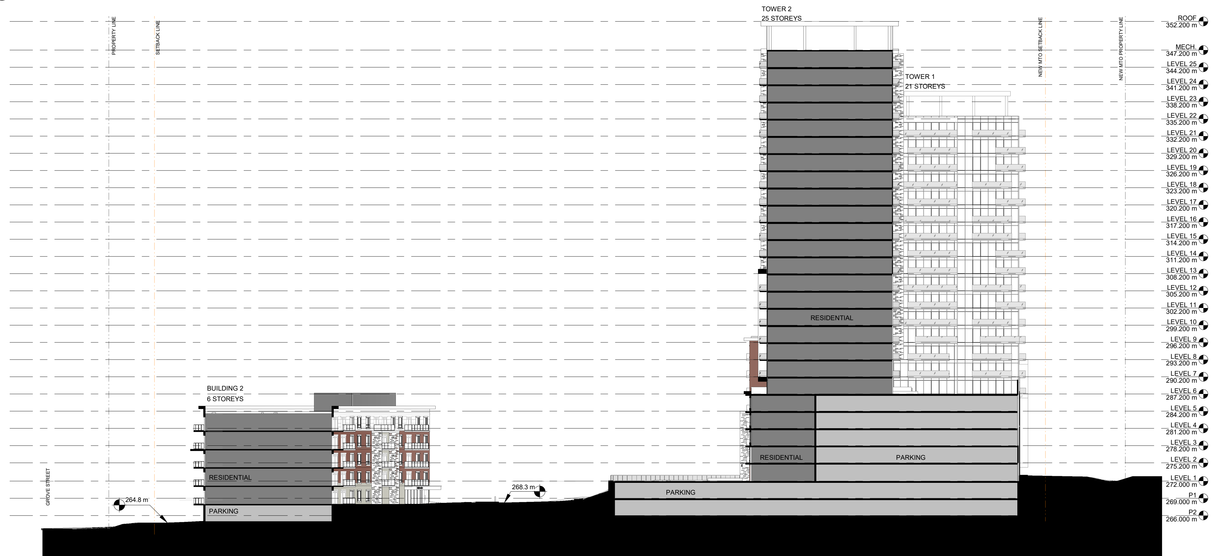
2 SITE SECTION 2 1:400
