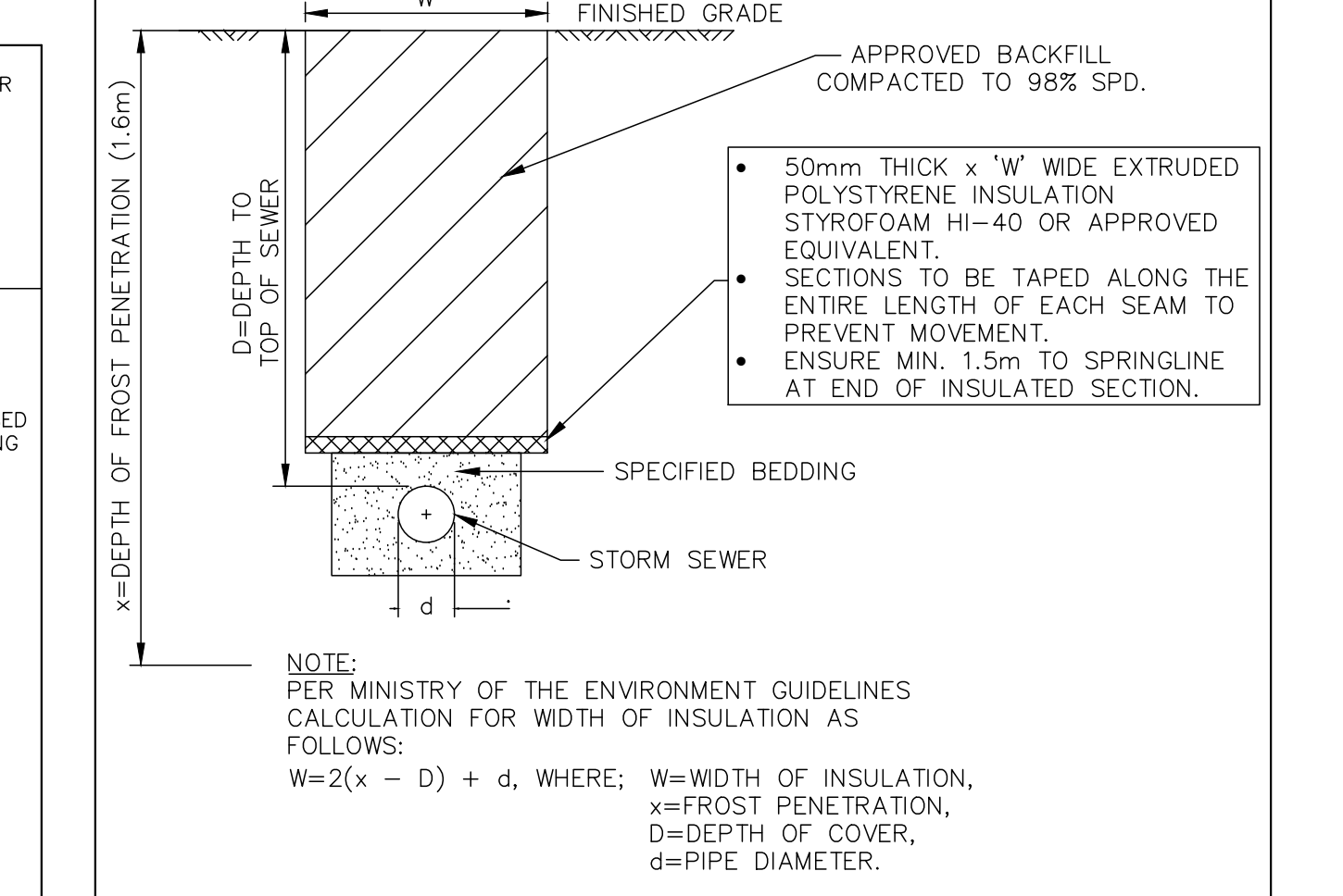
PIPE INSULATION DETAIL (N.T.S.)
